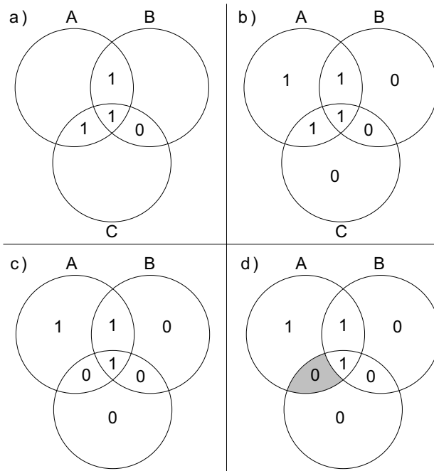
Slika 2: Hamingov kod za korekciju greške
