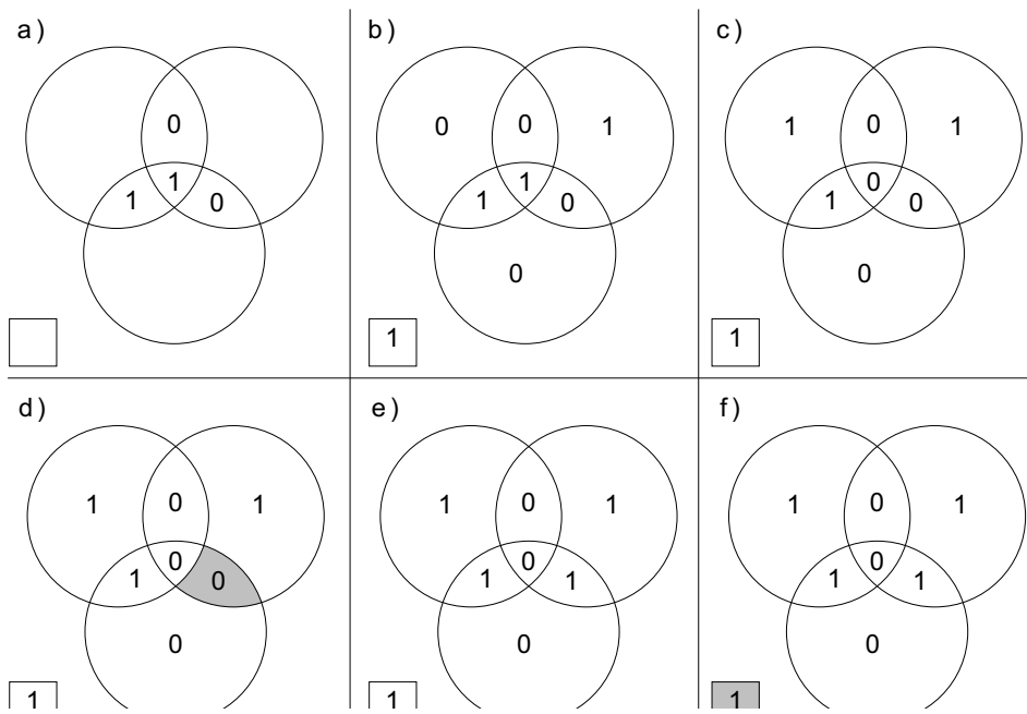
Slika 3: Hamingov SEC-DED kod
